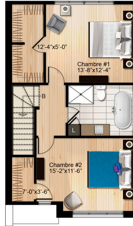
ÉTAGE 2 CH. 615 p.c.
